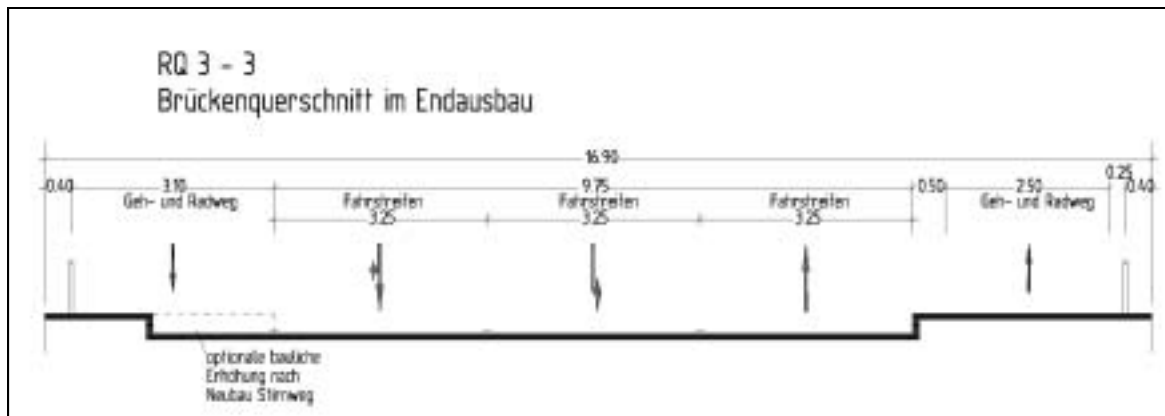
Abbildung 6: Szenario A.2.1, Brücke Hilpertstraße, Querschnitt
