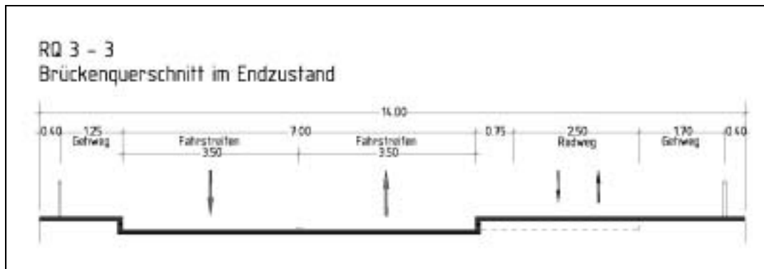
Abbildung 3: Szenario A, Stirnwegbrücke, Querschnitt
