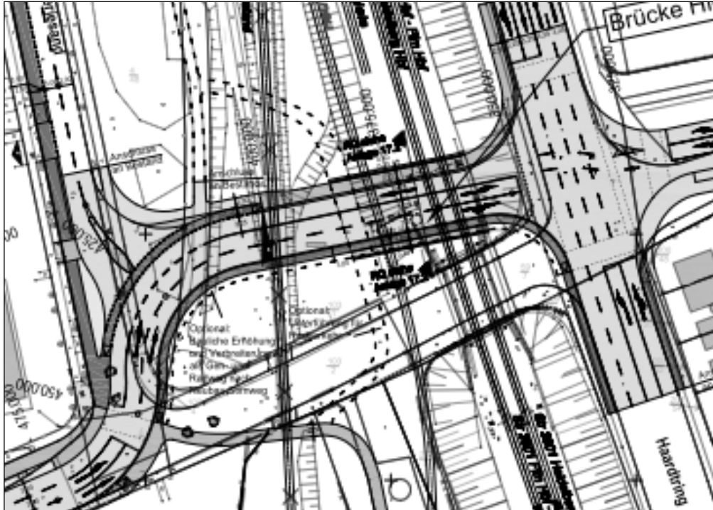
Abbildung 5: Szenario A.2.1, Brücke Hilpertstraße in Seitenlage, Vorfahrt geregelt
