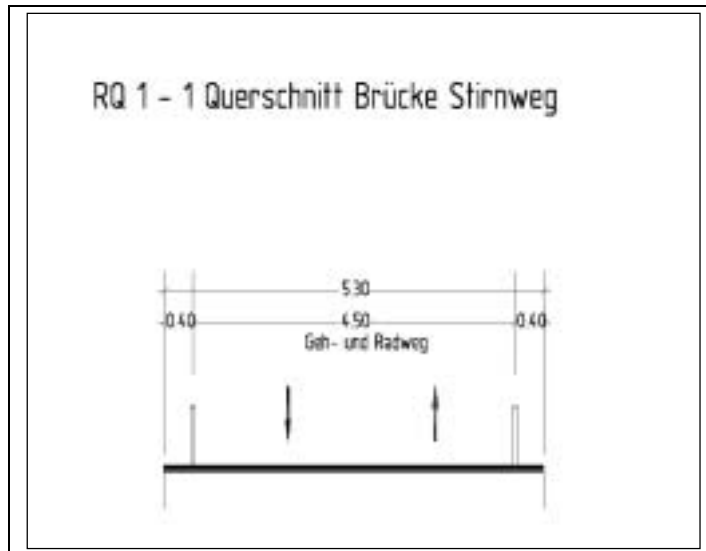
Abbildung 9: Szenario B, Stirnwegbrücke
