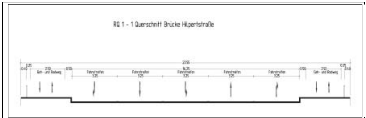
Abbildung 13: Szenario B.2, Brücke Hilpertstraße, Querschnitt
